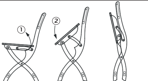
Сборка/Разборка стула
